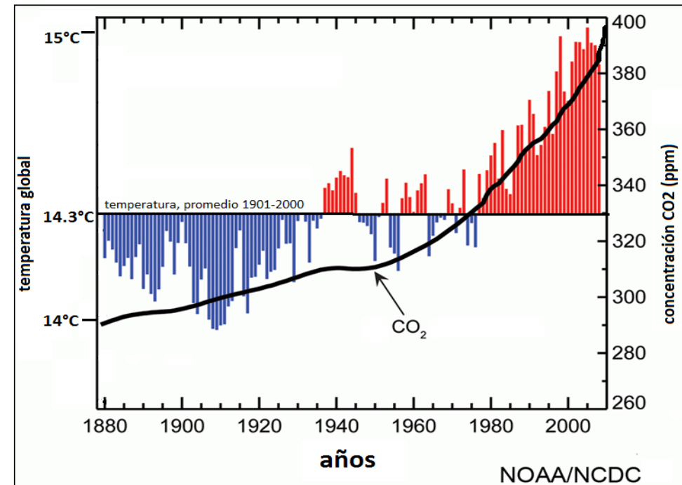
Temperatura y CO 2 en la atmósfera
