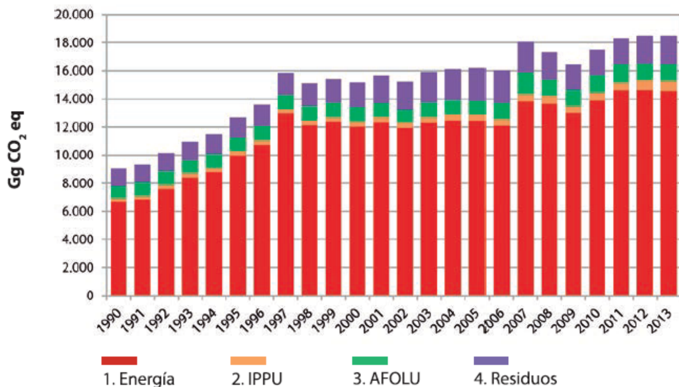
Figura 17. Metropolitana: emisiones y absorciones de GEI (Gg CO 2 eq) por sector, serie 1990-2013
