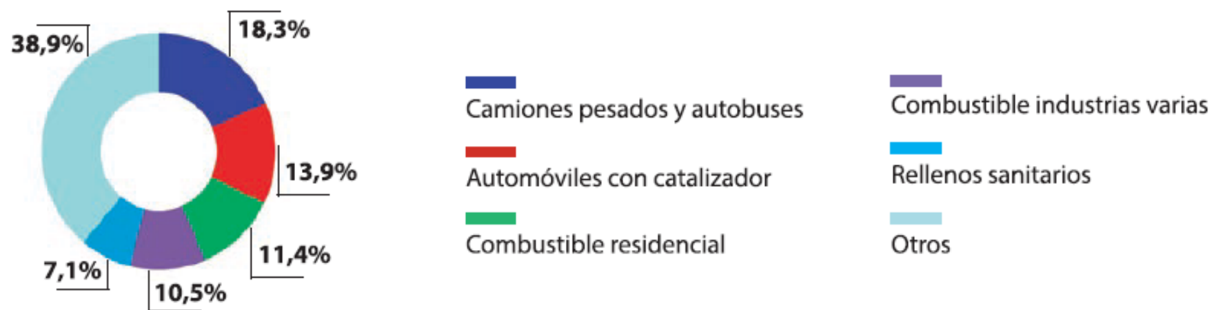
Figura 18. Metropolitana: principales fuentes y sumideros de GEI, año 2013
